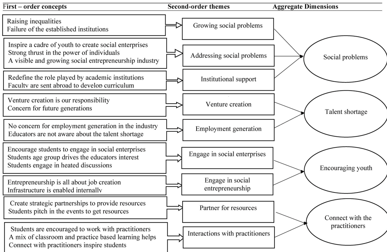
Fig. 1. Data analysis.
